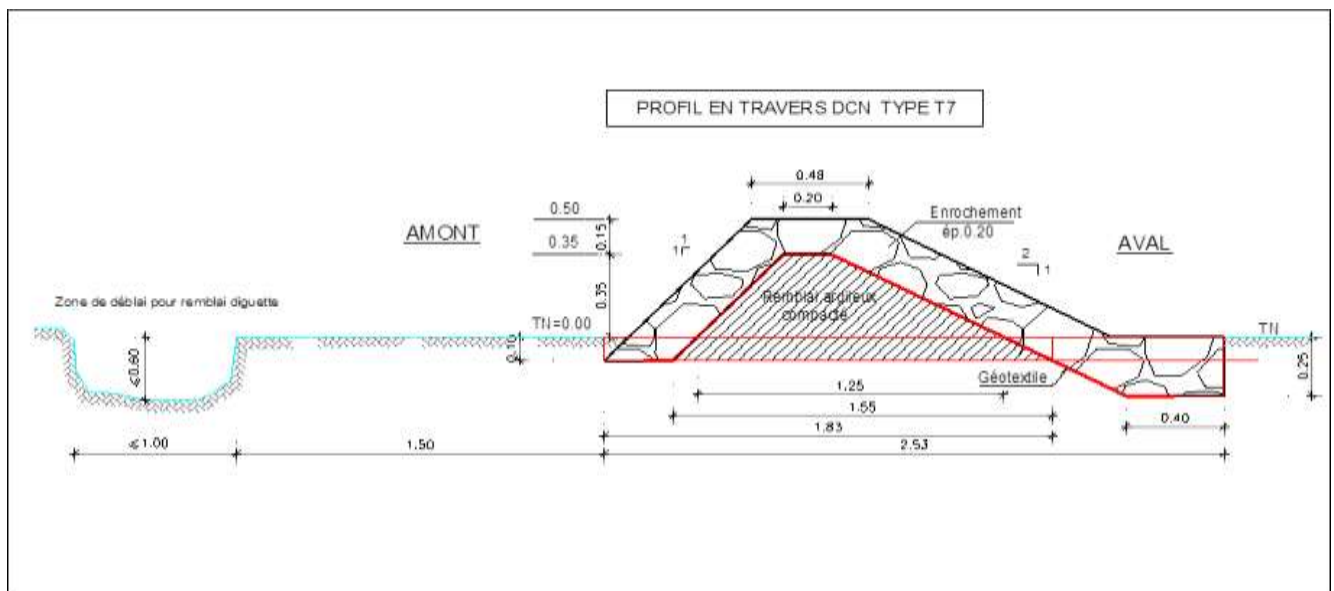
Figure 1: Profil en travers DCN type 17
