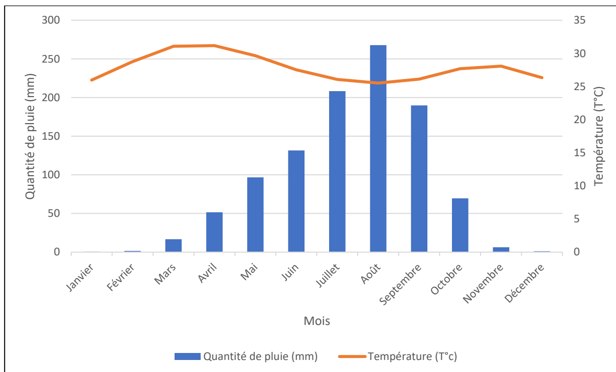
Graphique 1: Courbe ombrothermique de la station synoptique de Bobo-Dioulasso entre 1989-2019
